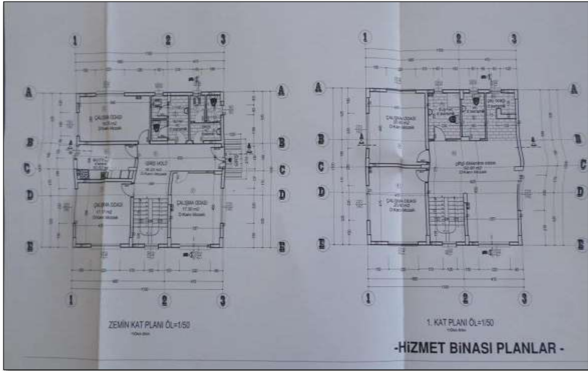
Hizmet Binası Planı
