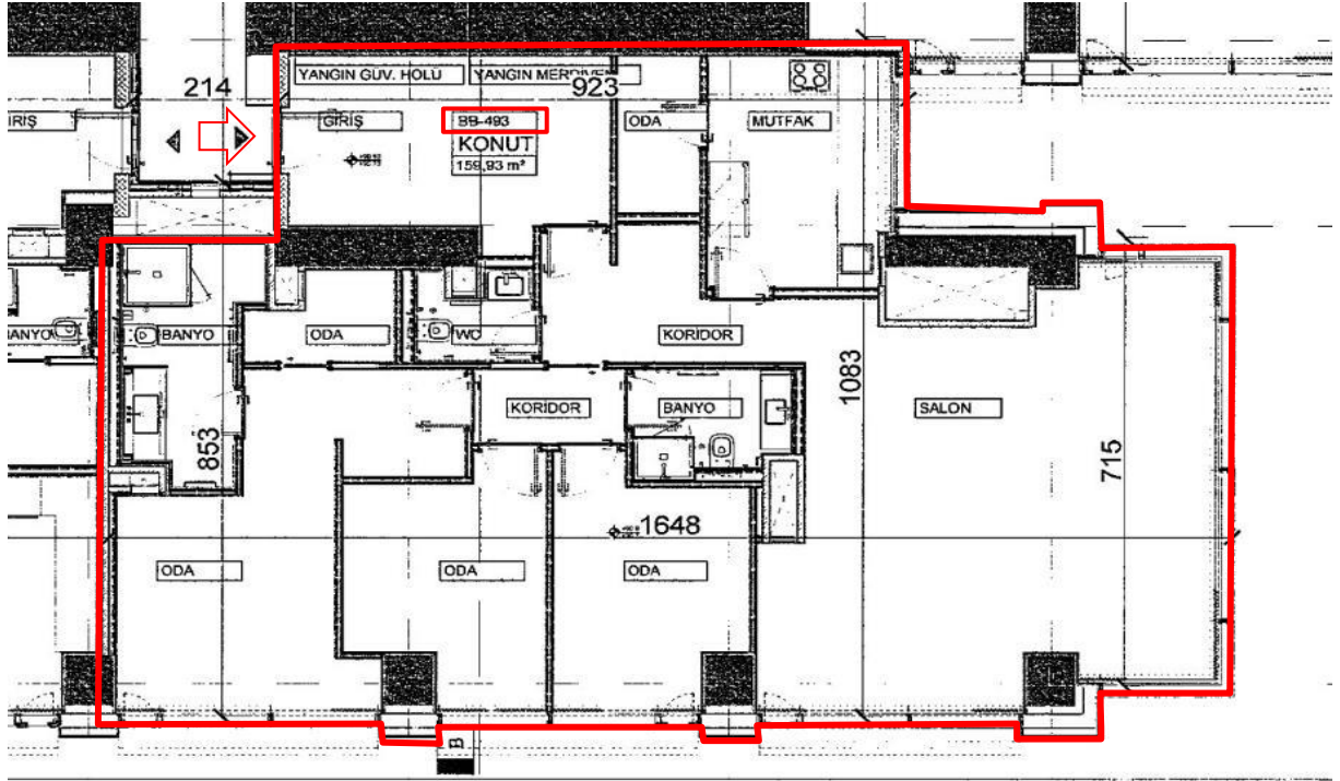
2. KULE 23. KAT 493 NOLU BB KAT PLANI
