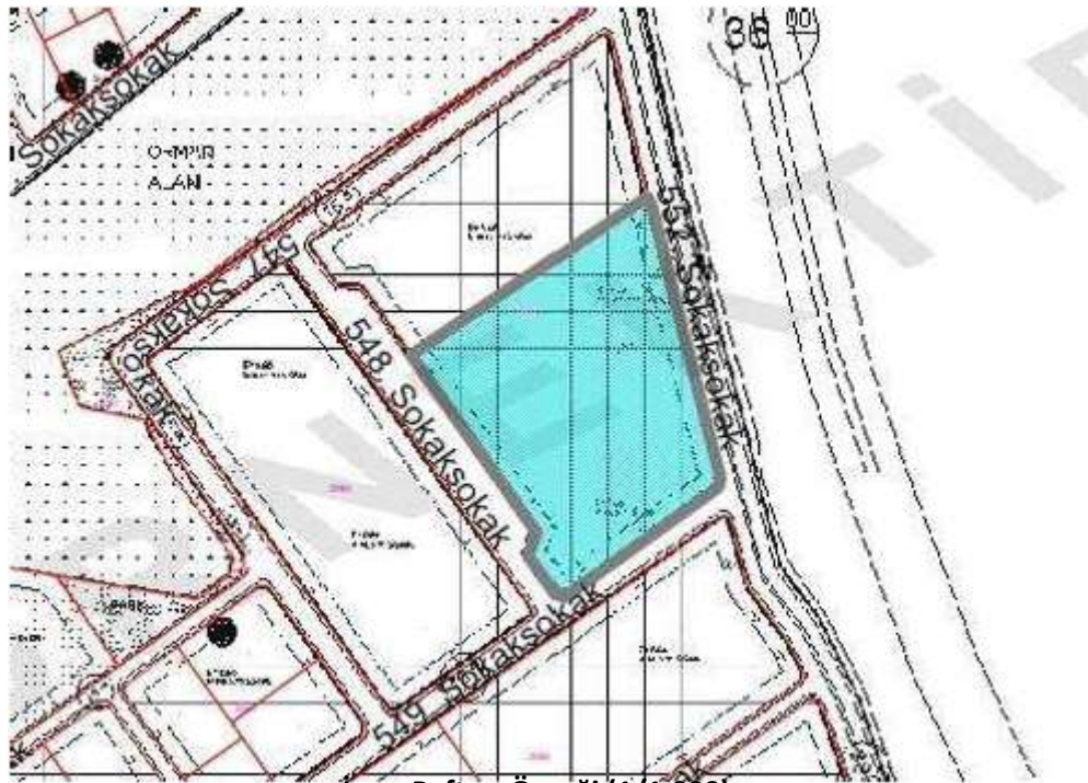
İmar Paftası Örneği (1/1.000)
